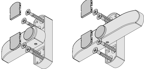
WSL 10 einflügelig
